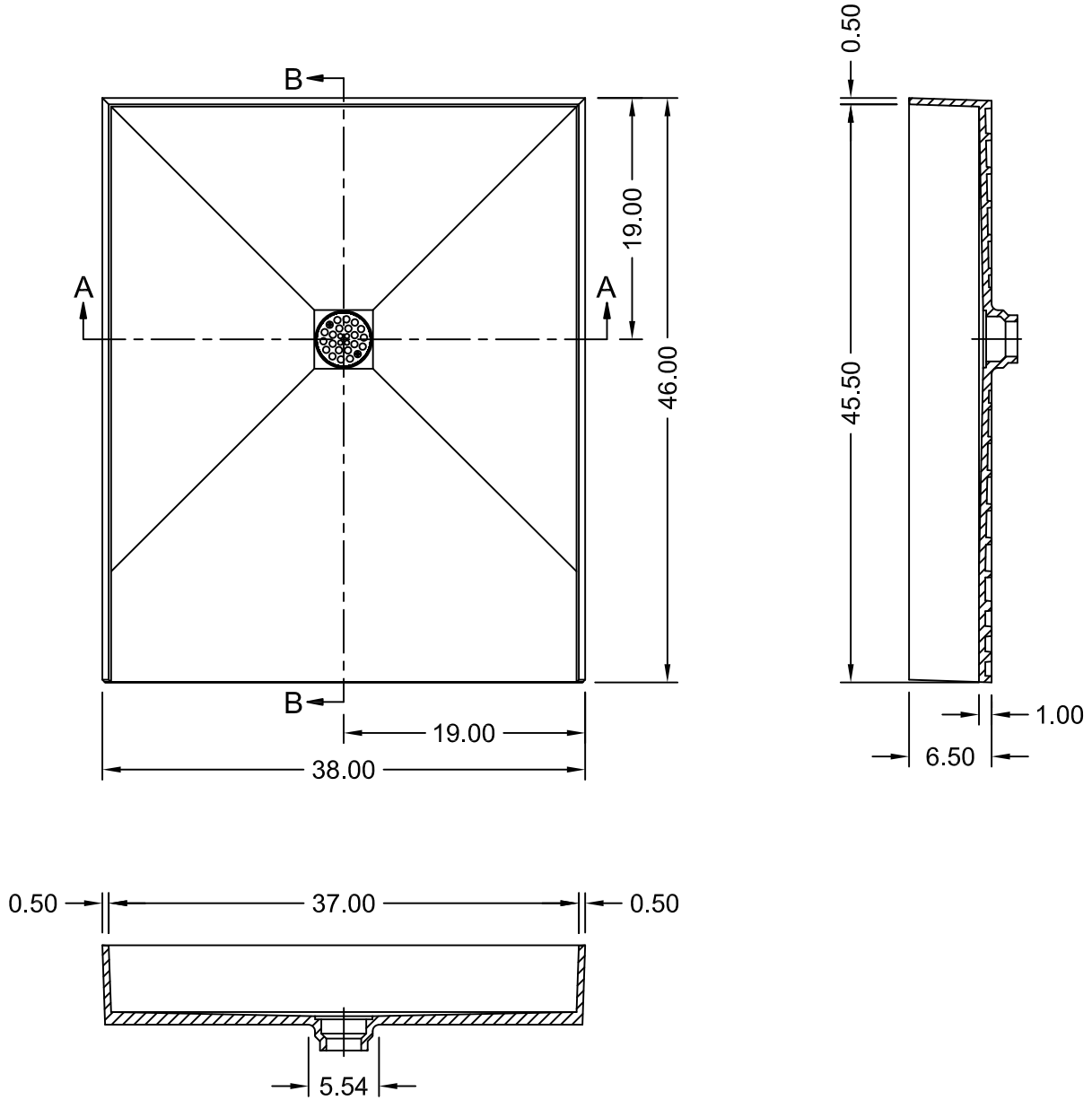
SECTION A-A
